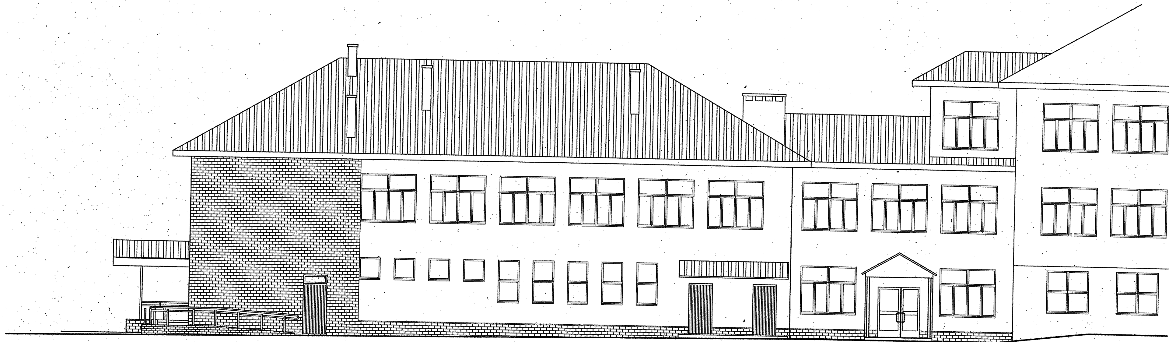
ELEWACJA POŁUDNIOWO-WSCHODNIA 1:100
